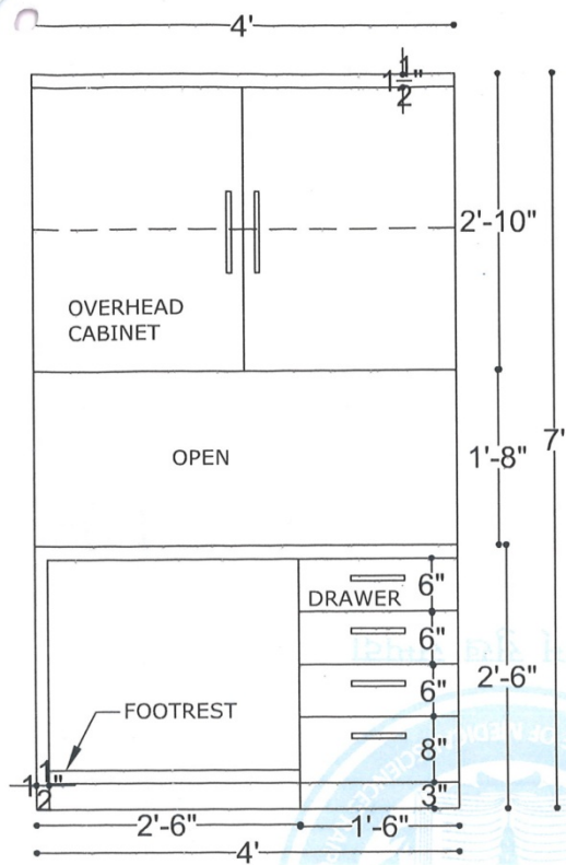
ELEVATION
